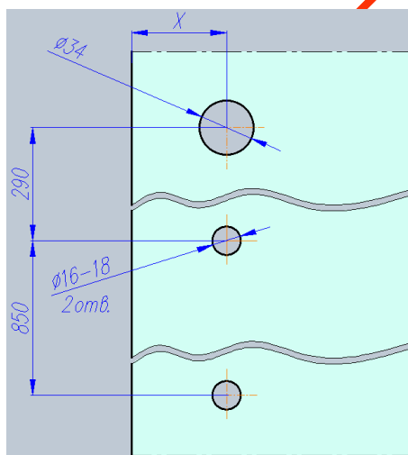
Вырез в стекле под OR-346_SSS
