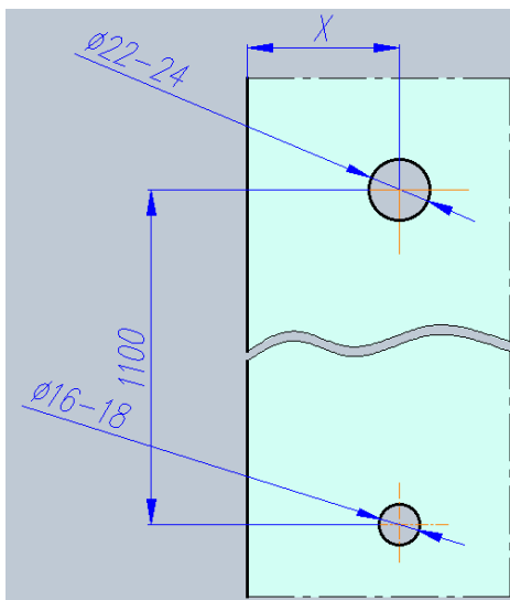
Вырез в стекле под OR-347.1500_SSS
